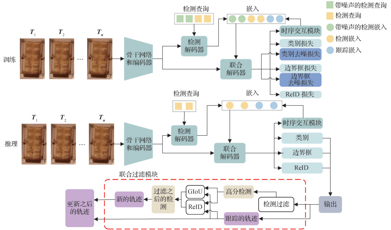
图1 DN-MeMOTR网络结构图
